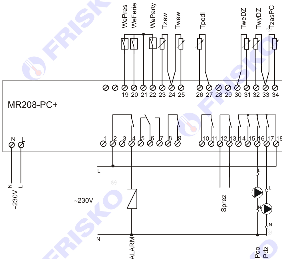
Schemat połączeń elektrycznych dla Układu:U1 .
