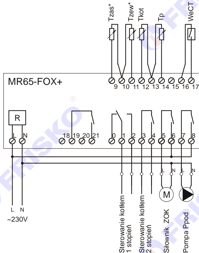
Schemat połączeń elektrycznych w układzie U2.
