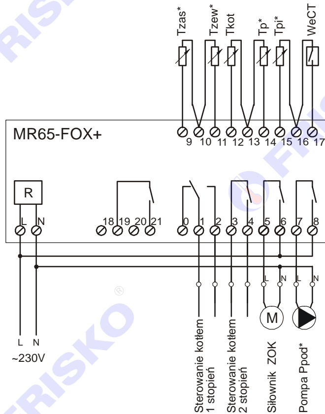
Schemat połączeń elektrycznych w układzie U1.
